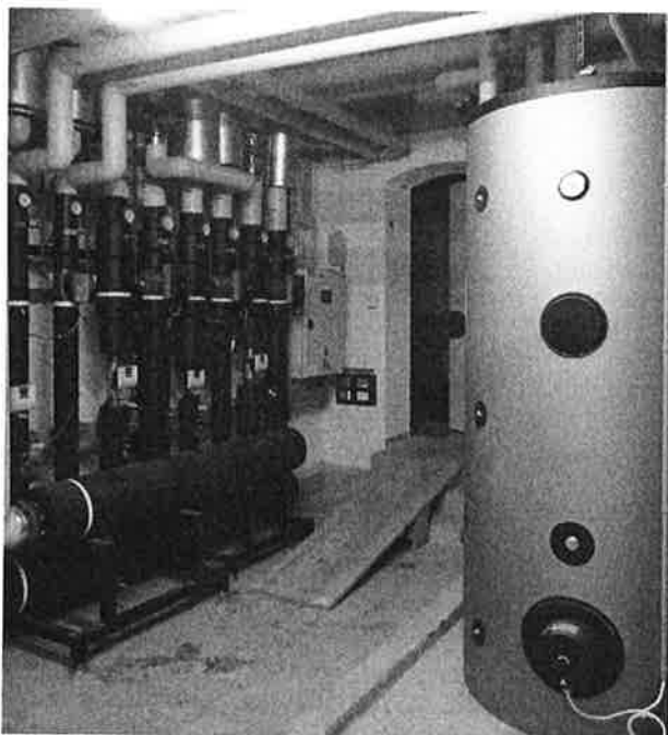
Neue Heizverteileranlage mit Warmwasserboiler
